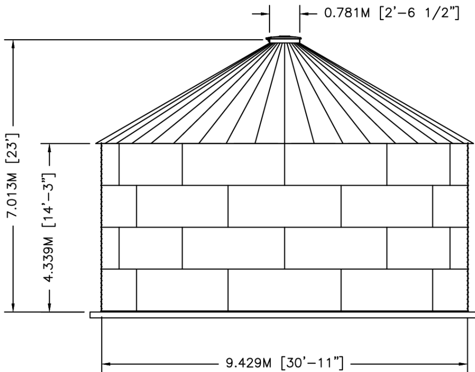
ELEVATION
